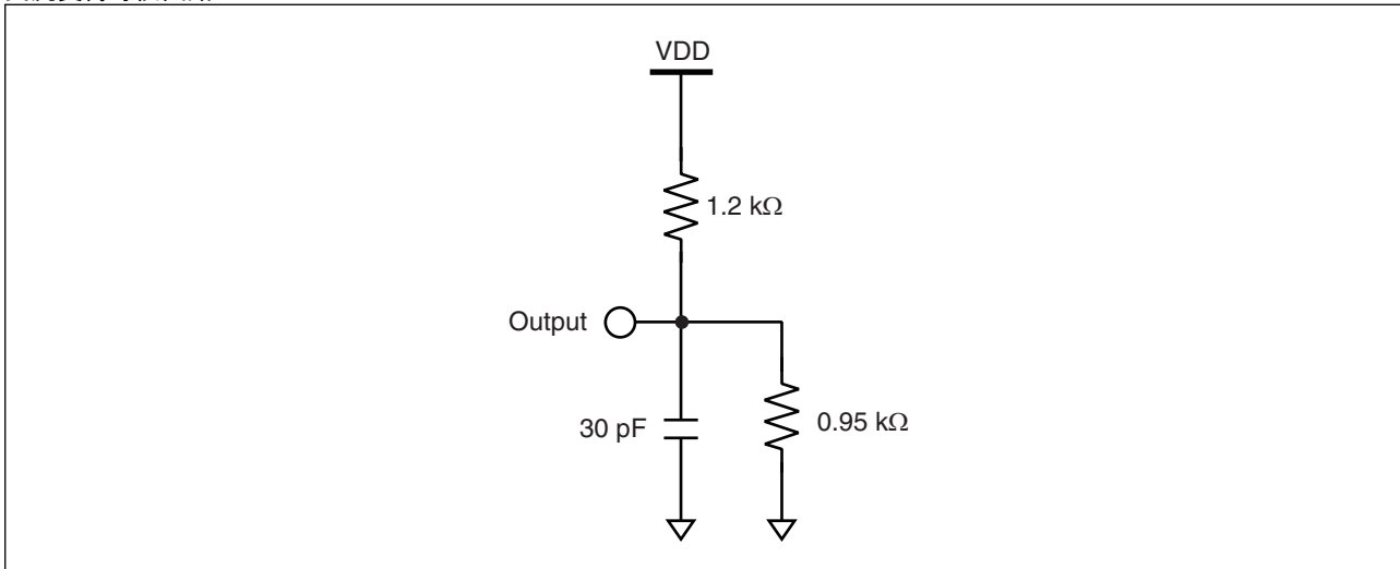
交流負荷等価回路 1
