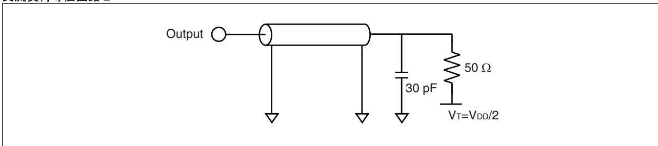
交流負荷等価回路 2
