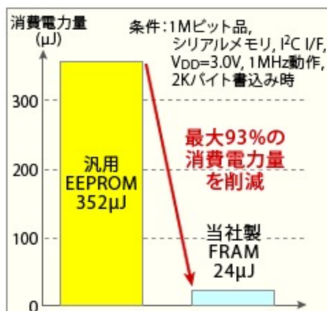
図2 消費電力比較(ライト時)
