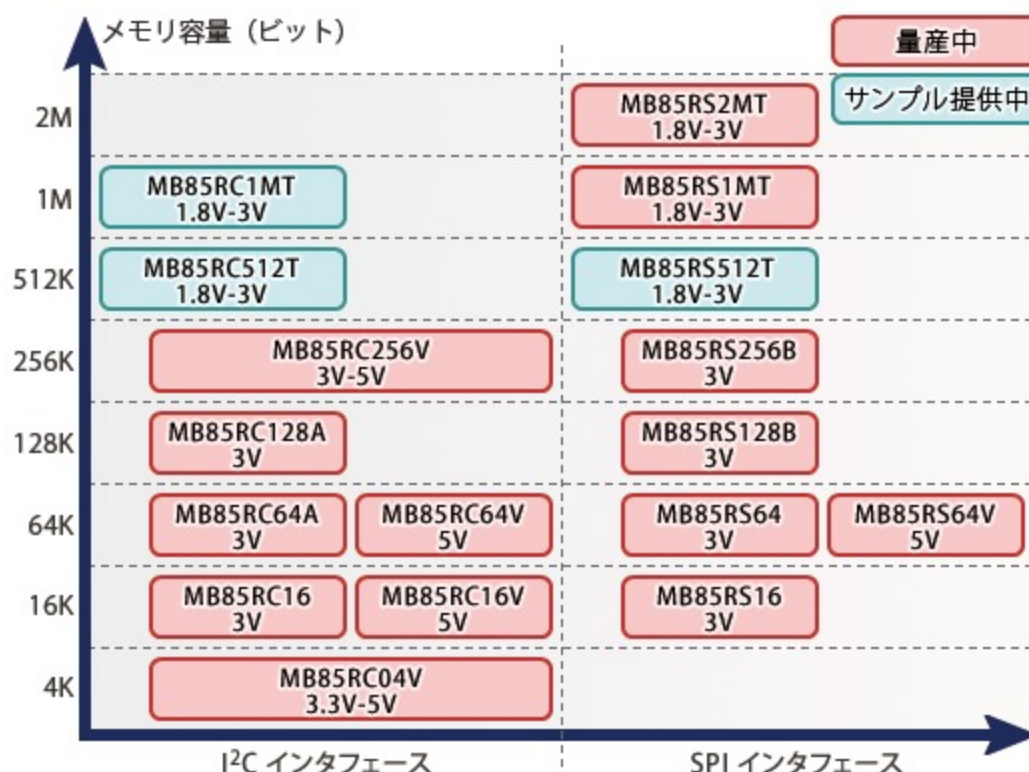
図3 FRAM製品のラインナップ(シリアルメモリ)
