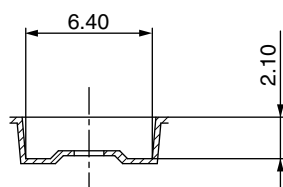
SEC.A-A
